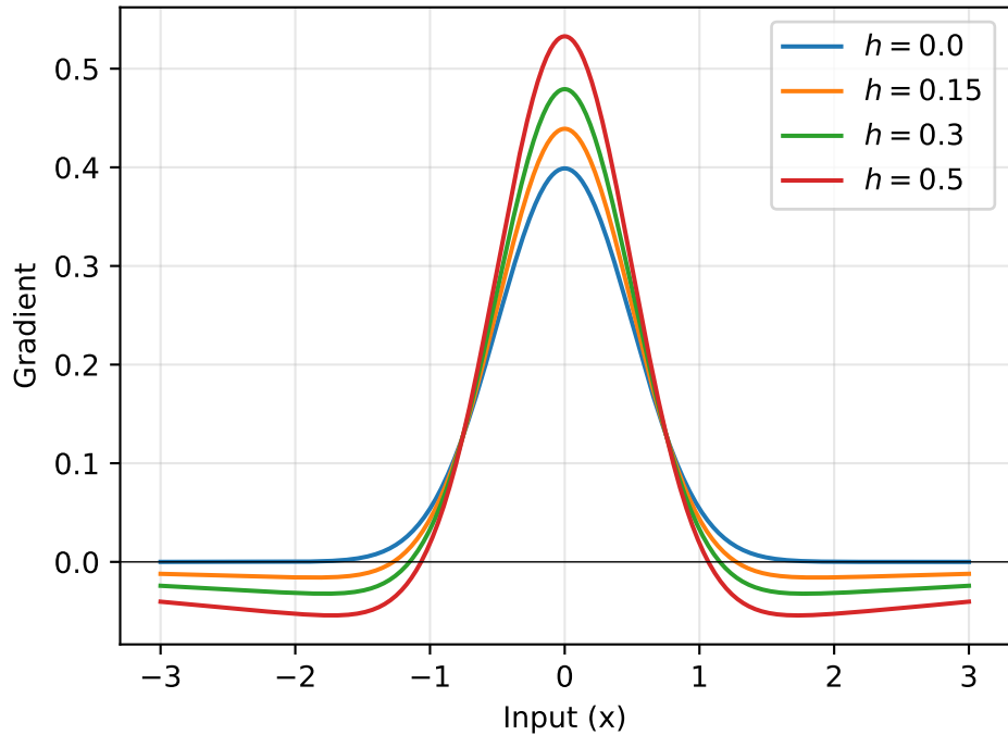
Effect of h Parameter
